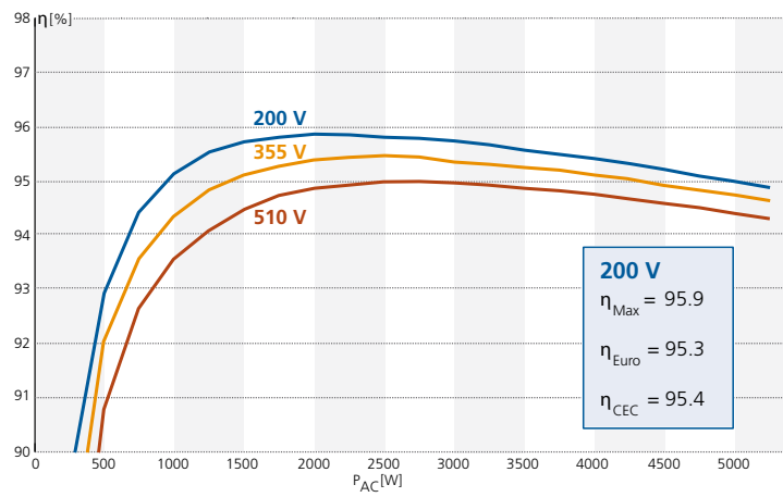
Wirkungsgradkennlinien Powador 6002
